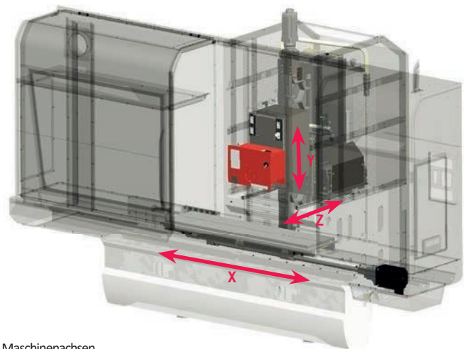
Maschinenachsen
